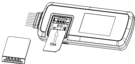
将 SIM 卡座防水硅胶垫片垫上
